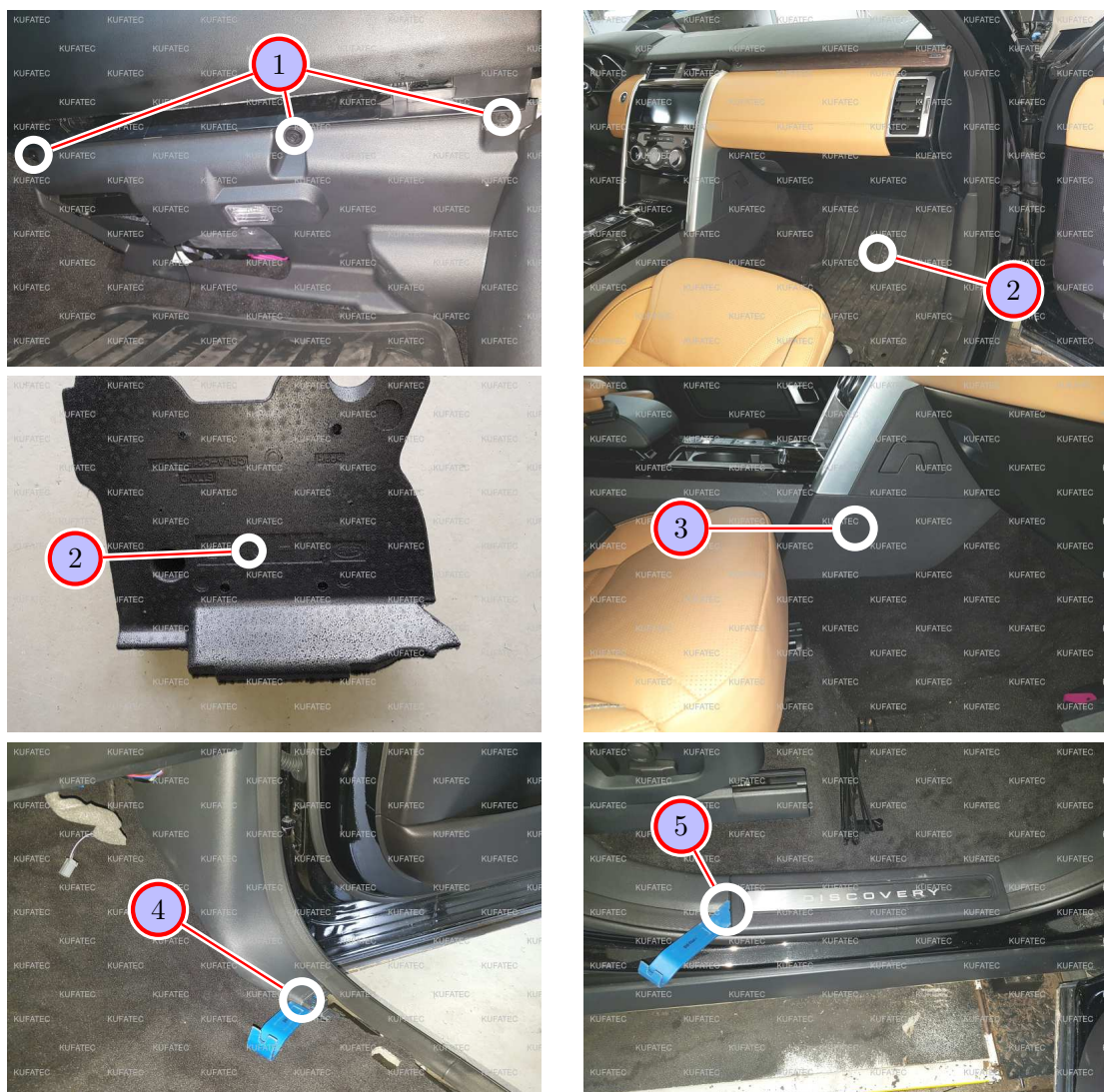
Figure 4: Demontage Verkleidungen Beifahrerseite
